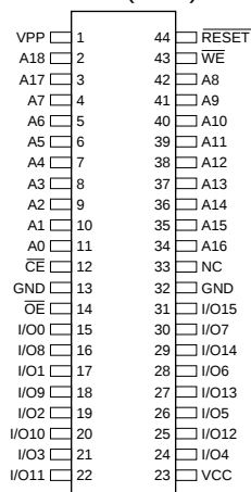
SOIC (SOP)
