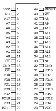
SOIC (SOP)
