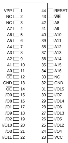
SOIC (SOP)
