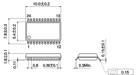
SSOP-A24
