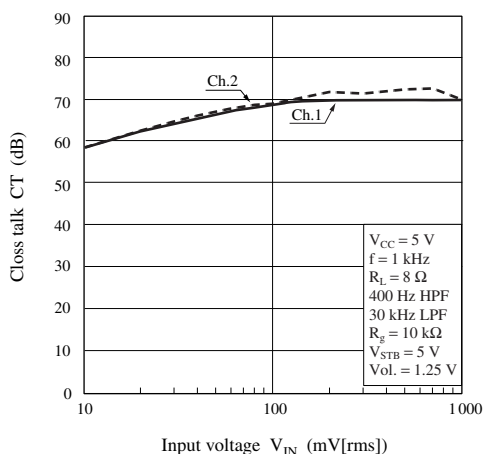
CT — V_{IN}
