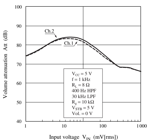
\text{Att} - V_{IN}
