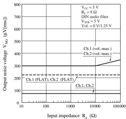
V_{NO} - R_g
