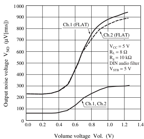
V_{NO} - \text{Vol.}
