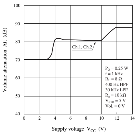
\text{Att} - V_{CC}
