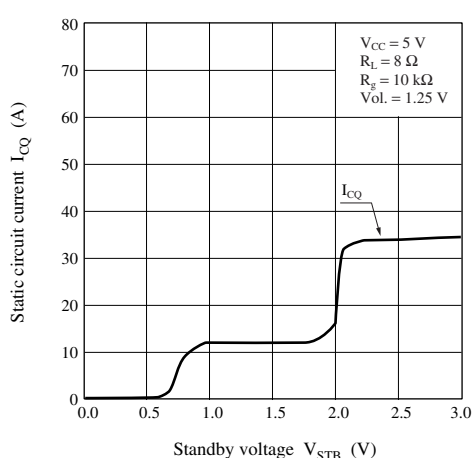
I_{CQ} - V_{STB}
