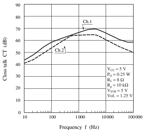
CT — f
