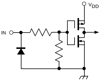
Dwg. EP-010-12
