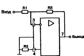
Конструктивные способы уменьшения токов утечки
