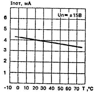
Зависимость тока потребления от температуры окружающей среды
