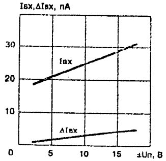
Зависимости входного тока и разности входных токов от напряжения питания
