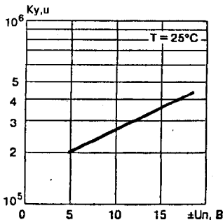
Зависимость коэффициента усиления напряжения от напряжения питания
