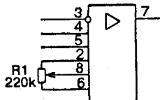
Схема внешней балансировки напряжения смещения
