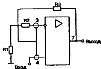
Возможные варианты соединения защитного кольца в базовых схемах включения ОУ
